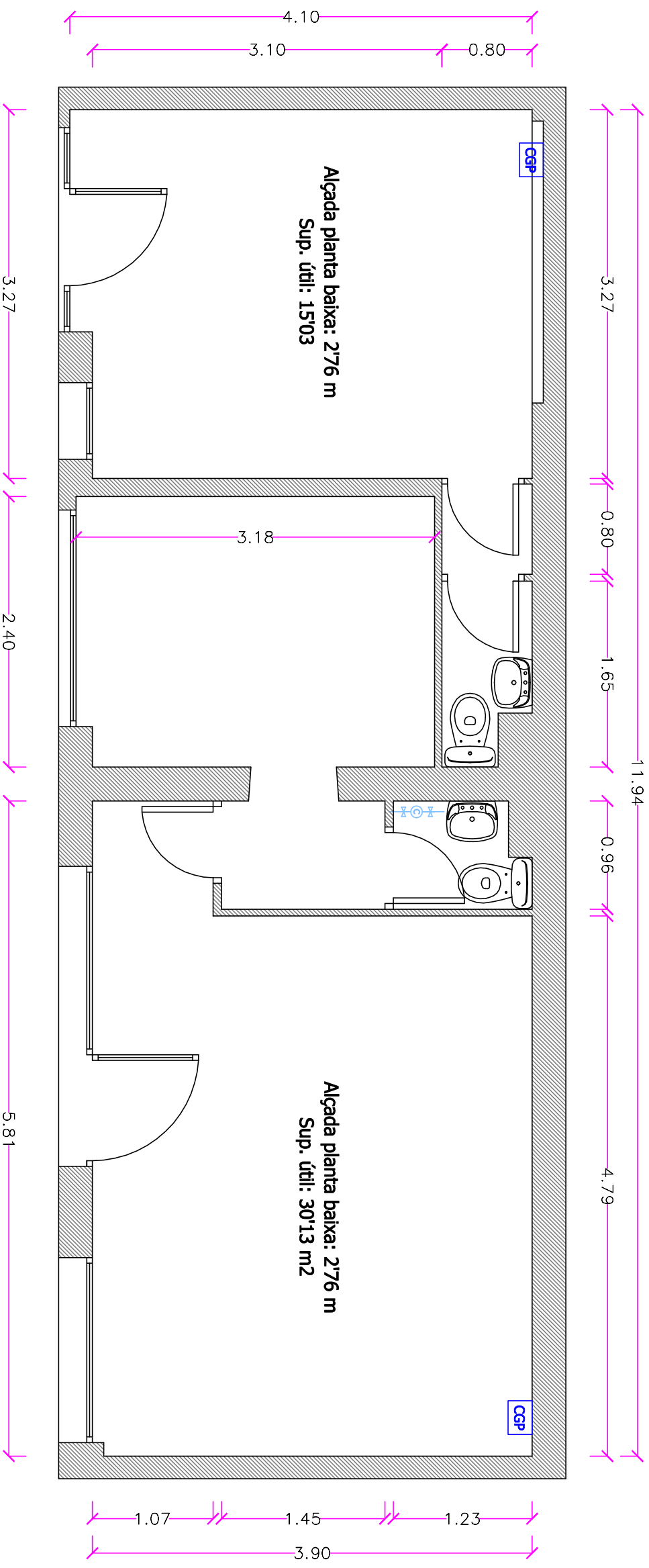
Planta Baixa L98 (Carrer La Manxa 15)
